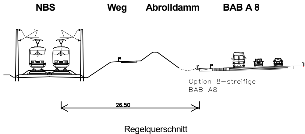
Abb. 1: Regelquerschnitt Bündelung BAB A8 – [NBS]
