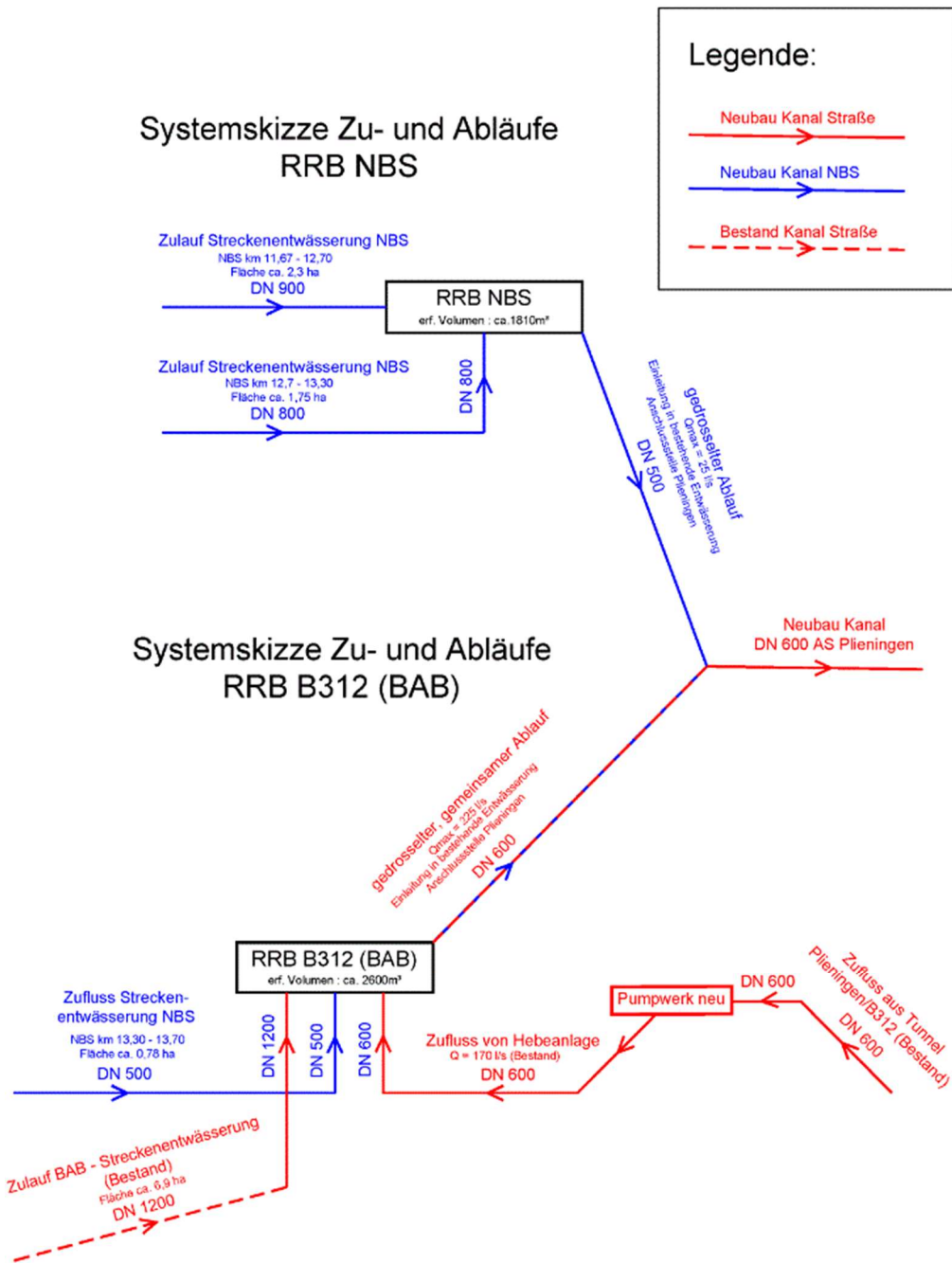
Abb. 14: Systemskizze der Zu- und Abläufe zu den RRB (Die blauen Anteile der Schemazeichnung ist eine zeichnerisch gewählte Darstellung aus der Ursprungsunterlage. Diese blaue Darstellung ist kein Inhalt von Planänderungen)
