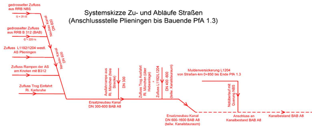
Abb.15: Systemskizze der Zu- und Abläufe für AS Plieningen bis Bauende PFA 1.3a (Die blauen Anteile der Schemazeichnung ist eine zeichnerisch gewählte Darstellung aus der Ursprungsunterlage. Diese blaue Darstellung ist kein Inhalt von Planänderungen)
