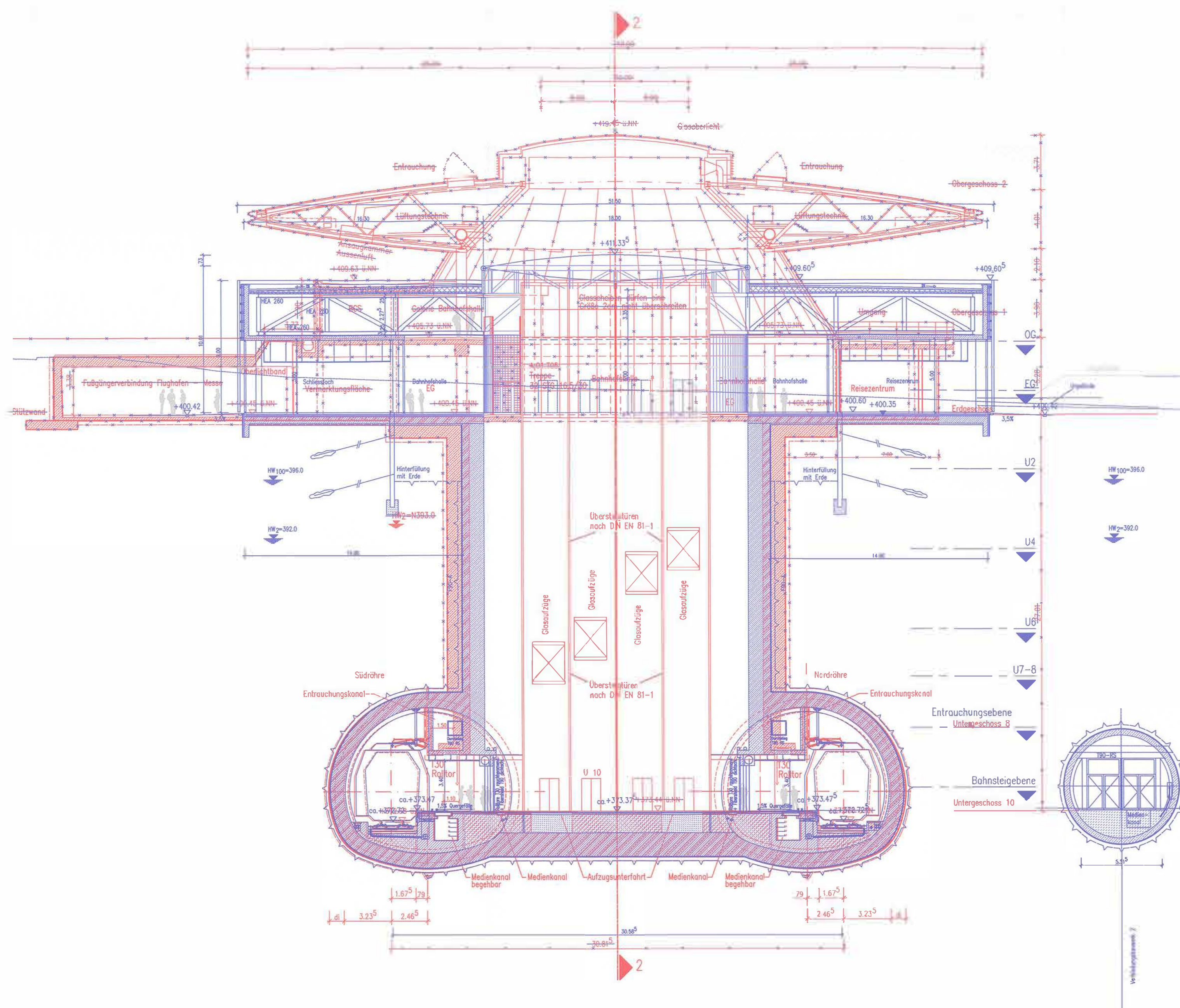
Schnitt 1-1 M 1:200
