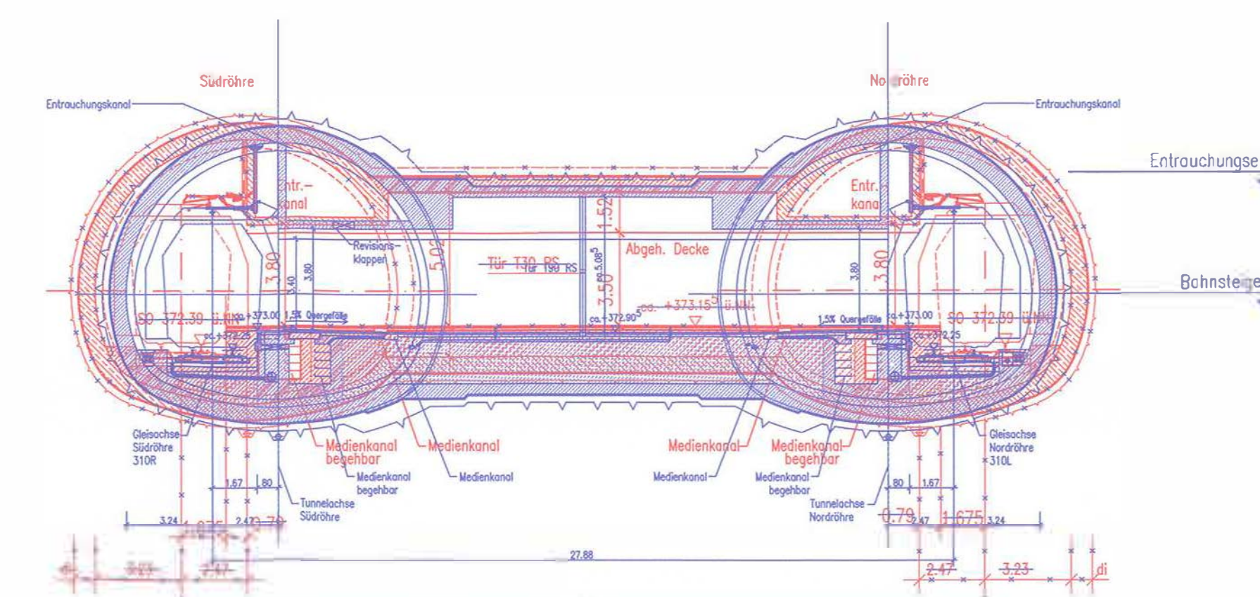
Schnitt Verbindungsbauwerk 4 M 1:200
