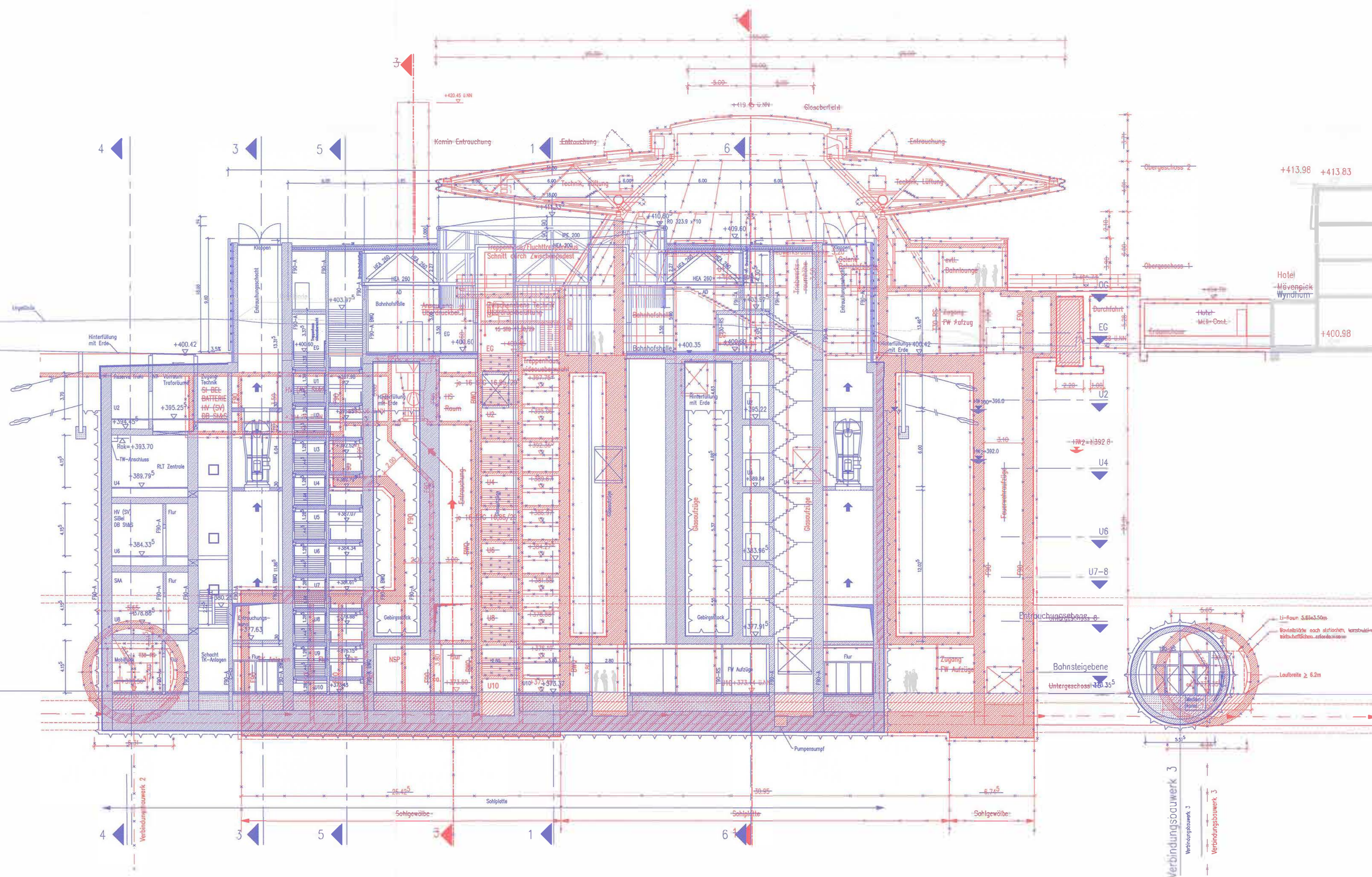
Schnitt 2-2 M 1:200
