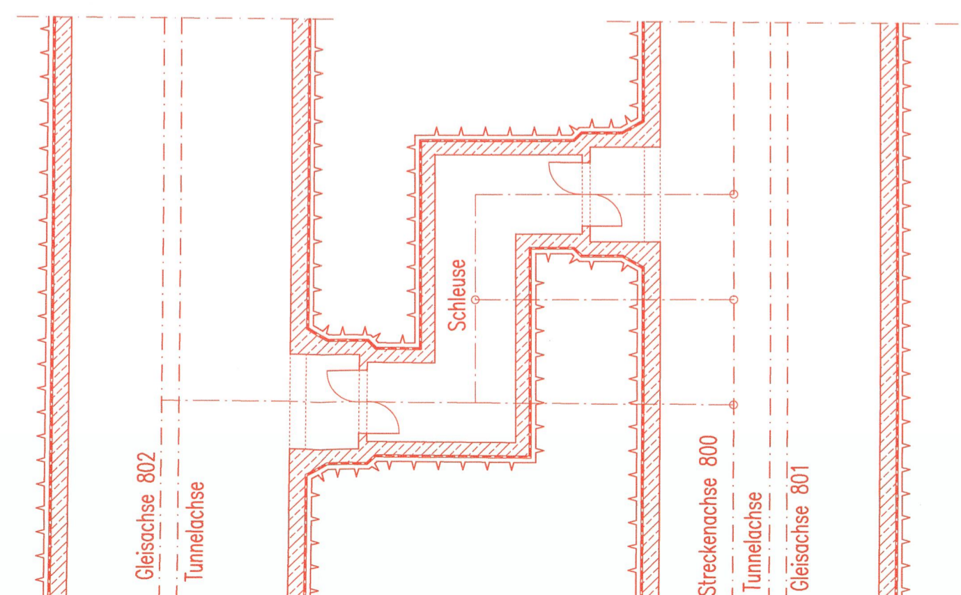
Grundriss Verbindungsbauewerk Sonderlösung 1, 8, 8a, 9 und 9a
