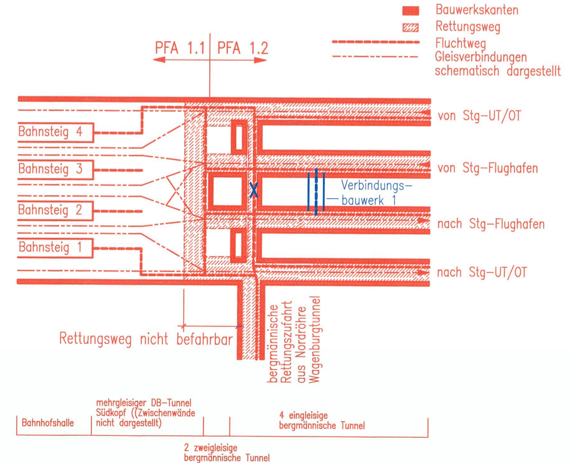
Systemskizze Flucht- und Rettungs-konzept DB-Tunnel Südkopf
