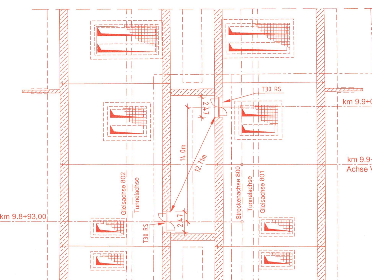
Grundriss Verbindungsbauewerk 10a
