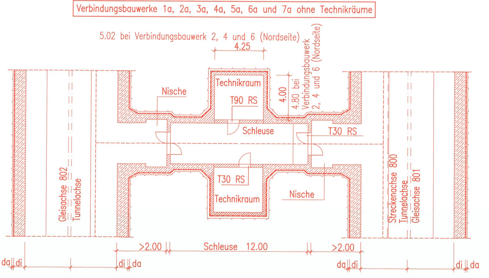
Grundriss Verbindungsbauewerk 1a-7a
