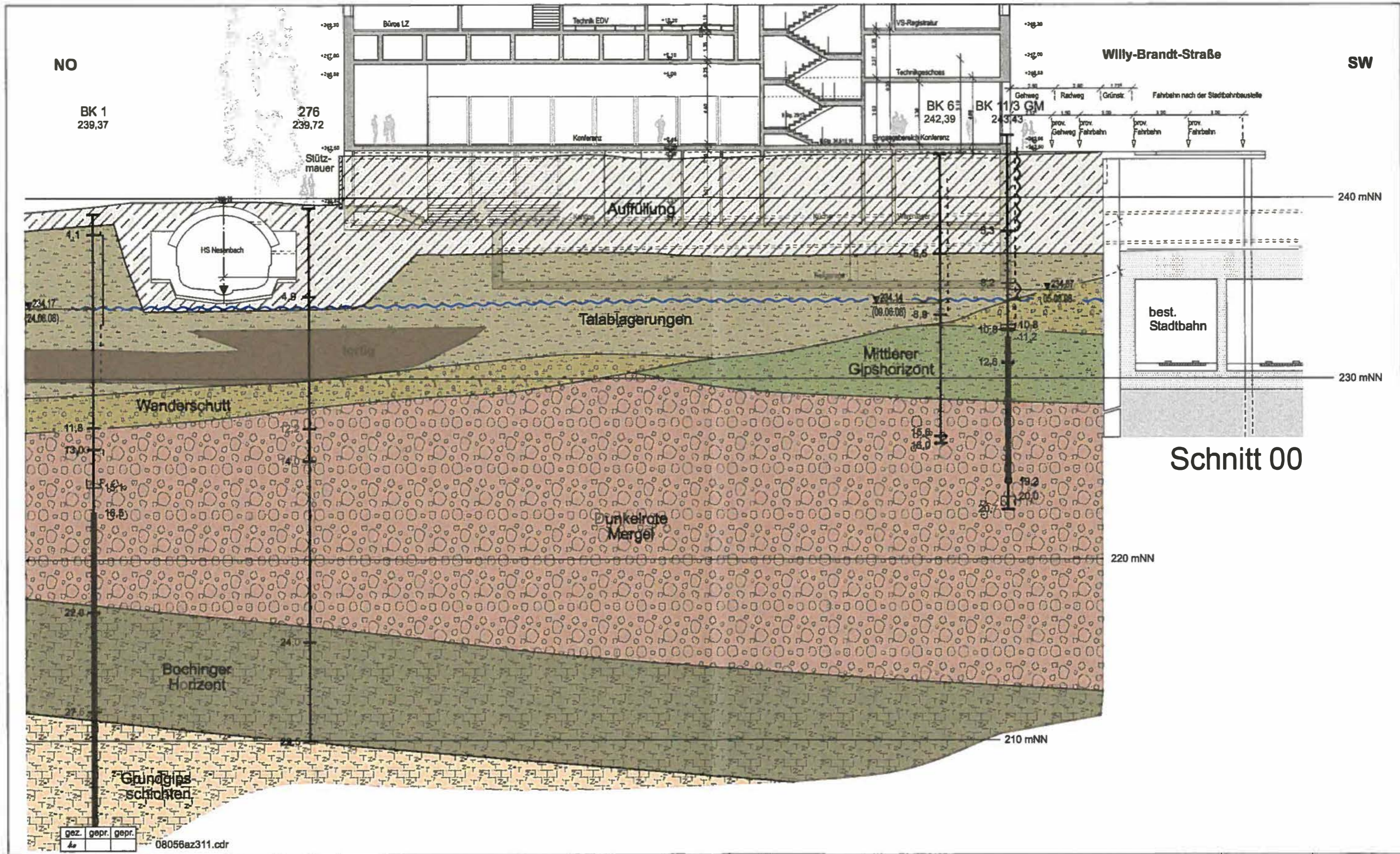
Geologischer Geländeschnitt C (Schnittführung siehe Anlage 1.2)
