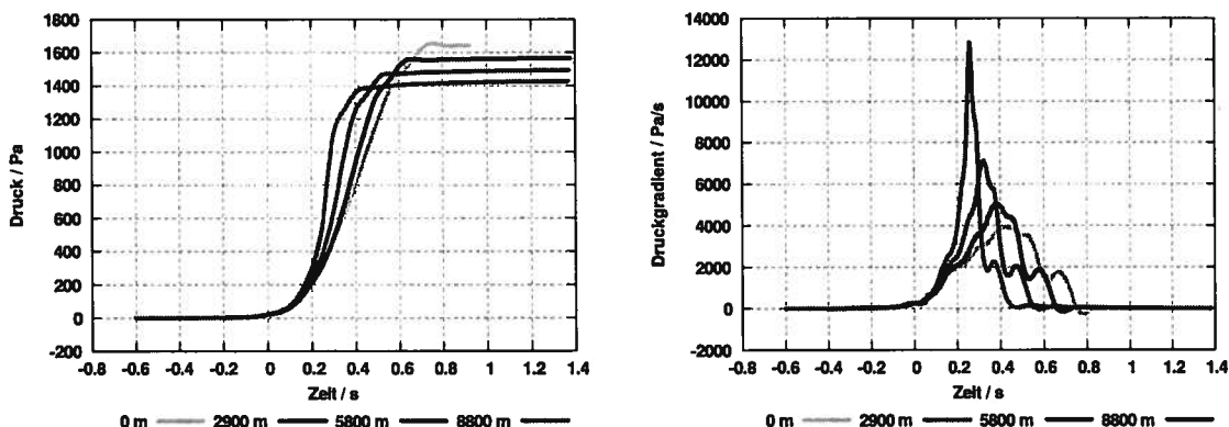
Bild 8: Aufsteilung der Druckwelle nach der Einfahrt eines TSI Zuges mit 250 km/h ins Portal Buch in verschiedenen Sektionen des Tunnels (links: Druck, rechts: Druckgradienten)
