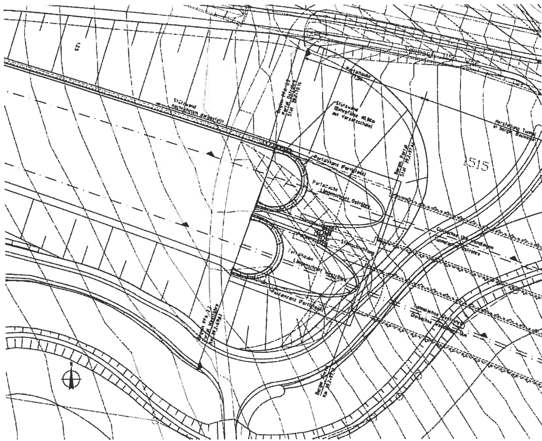
Anlage A2: Portal Aichelberg Portalansicht Quelle - „Anlage 8.3.8 Blatt 5 von 5 vom 13.03.2009“
