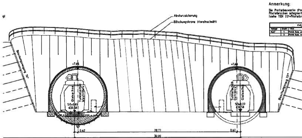
Anlage A5: Portal Buch Portalansicht Quelle - „Anlage 8.3.7 Blatt 6 von 6 vom 13.03.2009“
