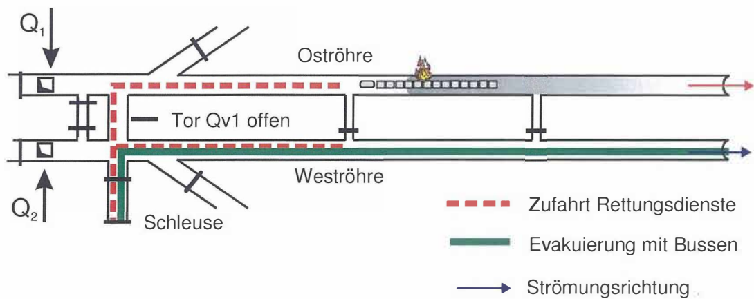
Abbildung 2: Fremdrettung bei einem Ereignis in der Oströhre
