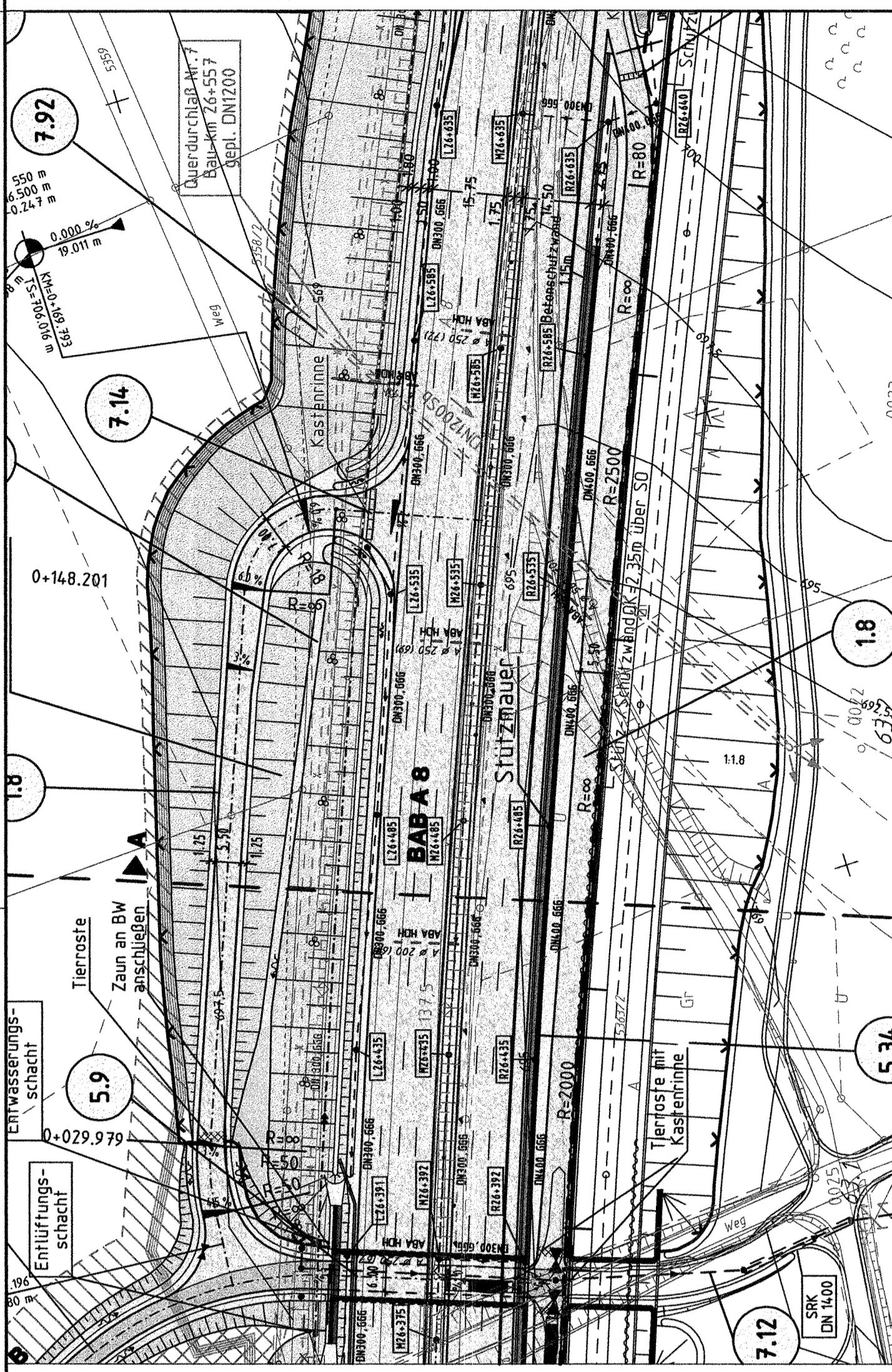
Lageplan M 1:1000
